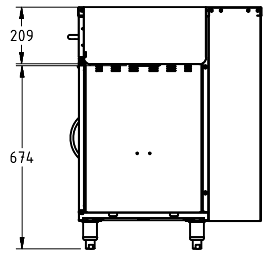
SECTION B-B ( 1 : 14 )
