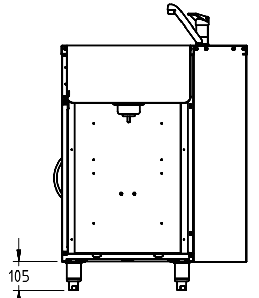
SECTION B-B ( 1 : 14 )
