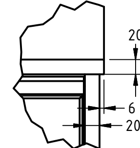
DETAIL B ( 1 : 5 )
